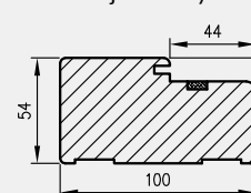
Przekrój poziomy ościeżnicy w murze
