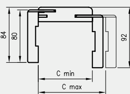
Przekrój TUN z ką. T80
