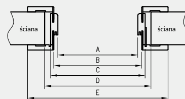
D - wymagana szerokość otworu w murze
