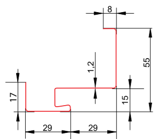
Ościeznica stalowa z uszczelką do drzwi stalowych technicznych 40 FD-21/N
